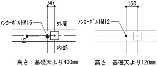
ホールダウン用アンカーボルト配置 アンカーボルト配置
